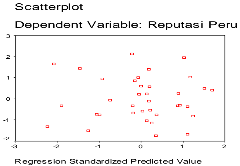
Gambar 5 Hasil Uji Heterokedastisitas Hipotesis 2
