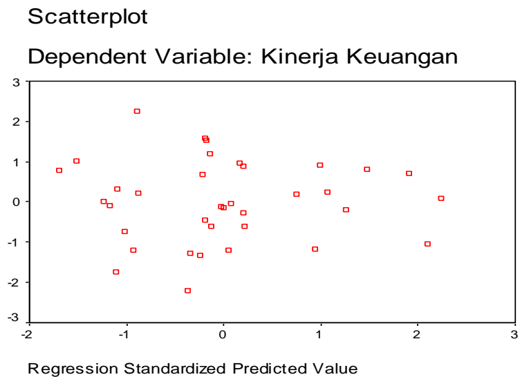
Gambar 5 Hasil Uji Heterokedastisitas Hipotesis 2
