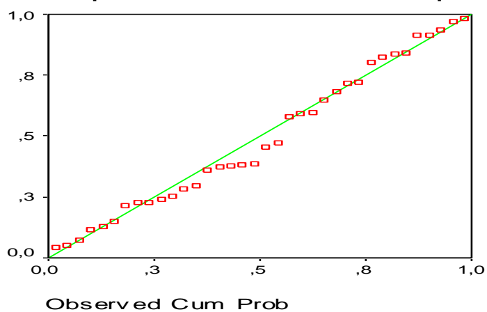
Gambar 3 Hasil Uji Normalitas Hipotesis 2
