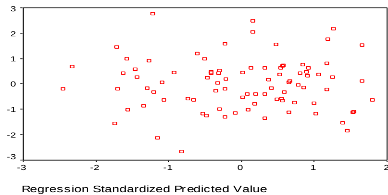
Gambar 4.2 : Grafik Scatter Plot
