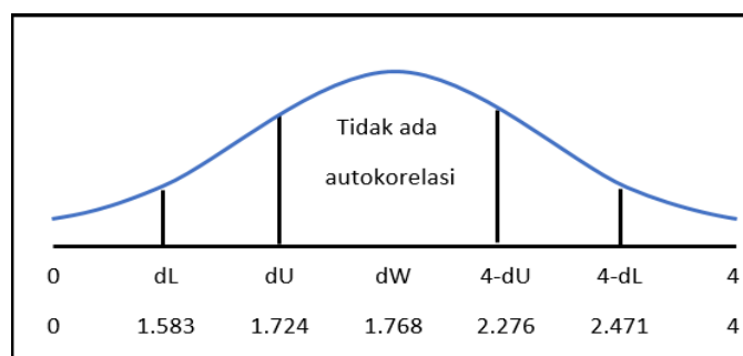
Gambar 4.1 : Kurva Uji Durbin Watson
