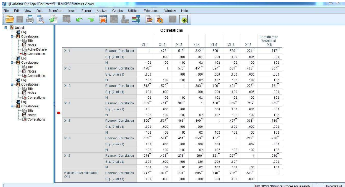
Gambar 1. Uji Validitas
